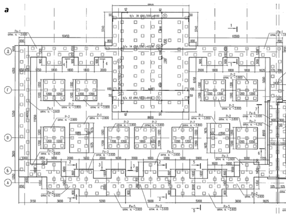
Рис. 3. Проектирование фундаментов
