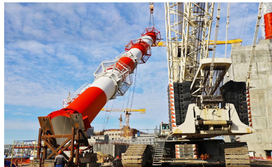
Курская АЭС. Монтаж вентиляционной трубы
